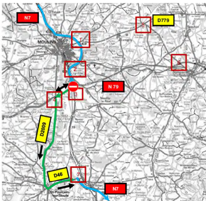
Itinéraire de déviation RN7 sens 1 PARIS → LYON
