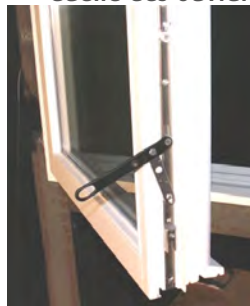
④ Fermeture individuelle des ouvrants
